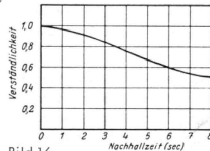
Bild 16 Verständlichkeit in Abhängigkeit von der Nachhallzeit
