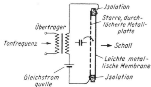
Bild 76 Schema und Anschaltung eines Kondensator-Lautsprechers
