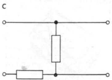
Bild 51 L-Glieder
