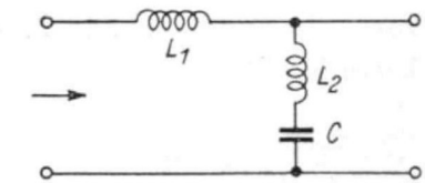
Bild 65 Tiefpaß mit 2 Drosseln
