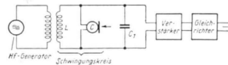
Bild 24 Hochfrequenzschaltung eines Mikrofons
