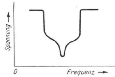
Bild 72 Frequenzkurve zum Bandpaß Bild 71
