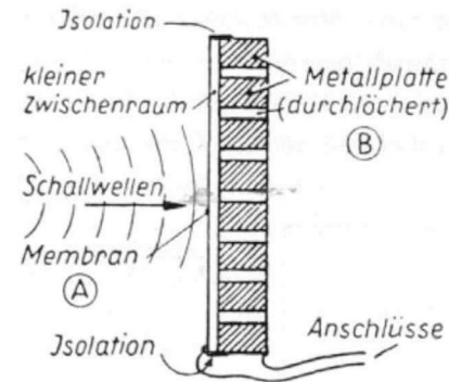
Bild 22 Schema eines Kondensator- Mikrofons (Schnitt)
