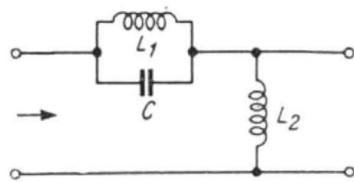
Bild 61 Hochpaß mit 2 Drosseln
