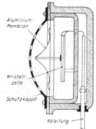
Bild 28 Schnitt durch ein Kristall- Membranmikrofon
