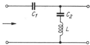
Bild 60 Hochpaß mit 2 Kondensatoren
