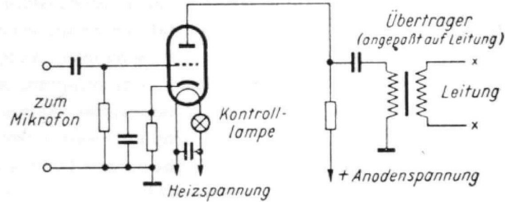
Bild 25 Schema eines Mikrofon- verstärkers
