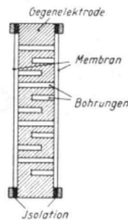
Bild 33 Kondensator-Mikrofon mit nierenförmiger Richtcharakteristik
