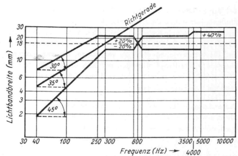
Bild 43 Zulässige Toleranzen einer Schallplattenaufnahmeapparatur gemessen durch die Lichtbandbreite
