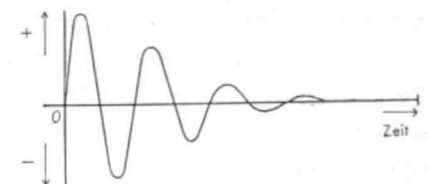
Bild 6 Gedämpfte Schwingungen
