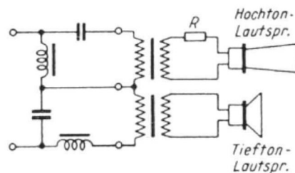
Bild 79 Lautsprecheranordnung mit elektrischer Weiche
