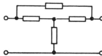
Bild 56 Überbrücktes T-Glied
