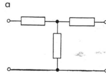
Bild 52 Unsymmetrische T-Glieder
