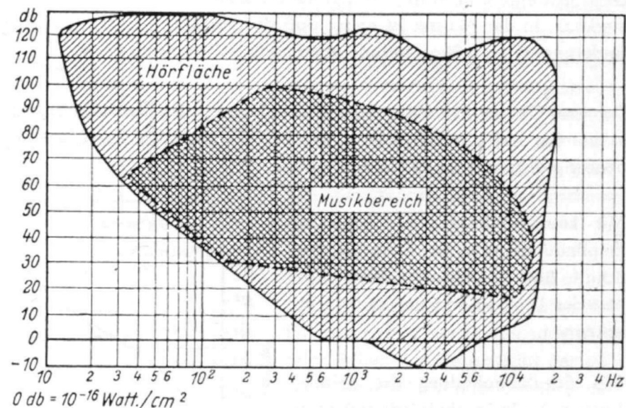
Bild 13 Umfang des Hörbereichs
