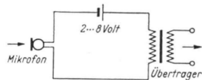
Bild 21 Schaltung eines Kontakt-Mikro- fons
