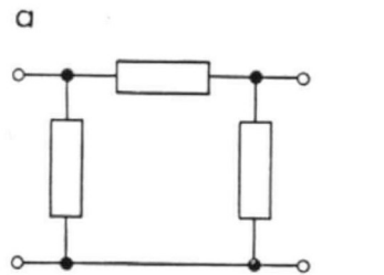
Bild 54 Unsymmetrische \pi -Glieder
