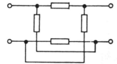
Bild 57 Kreuzglied
