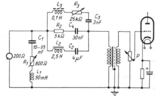
Bild 74 Filteranordnung für Ton- abnehmer (200 Ω)
