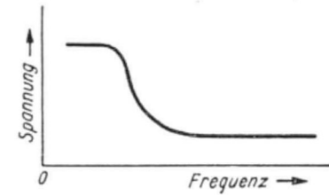
Bild 64 Frequenzkurve zu Paß Bild 63
