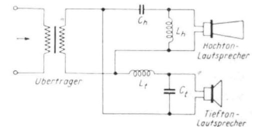
Bild 68 Hochpaß und Tiefpaß in Verbindung mit einem Hochton- und einem Tieftonlautsprecher
