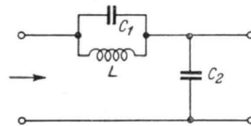
Bild 66 Tiefpaß mit 2 Kondensatoren
