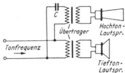
Bild 78 Möglichkeit der Anschaltung eines Hochton- und eines Tieftonlautsprechers
