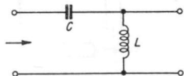
Bild 58 Grundsätzliche Form eines Hochpasses
