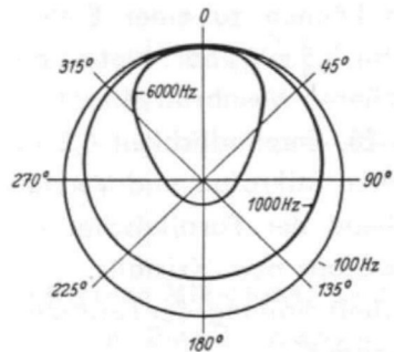
Bild 29 Richtwirkungskurven eines Mikrofons bei verschiedenen Frequenzen
