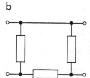
Bild 55 Symmetrisches \pi -Glied
