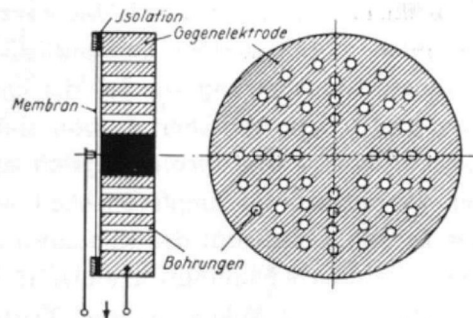
Bild 30 Kapsel eines Kondensator-Mikrofons (schematisch) mit Achtercharakteristik
