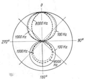
Bild 31 Richtcharakteristik des Mikrofons nach Bild 30
