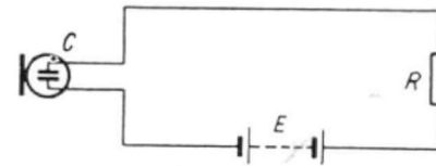
Bild 23 Schaltung eines Kondensator- Mikrofons
