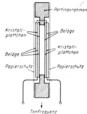
Bild 27 Schema der Klangzelle eines piezoelektrischen Mikrofons
