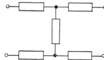
Bild 53 Symmetrisches T-Glied
