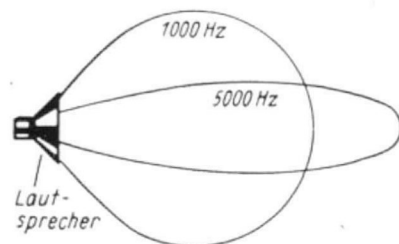
Bild 77 Die höheren Tonfrequenzen werden anders abgestrahlt als die niedrigen
