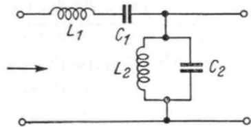
Bild 69 Schema eines Bandpasses (grundsätzliche Anordnung)
