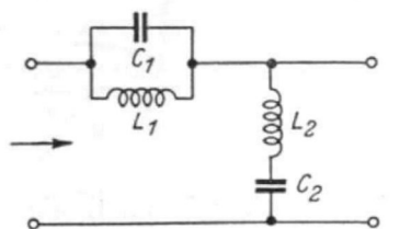
Bild 71 Bandpaß zur Unterdrückung eines bestimmten Frequenz- bandes
