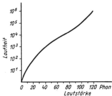
Bild 14 Abhängigkeit der Lautheit von der Lautstärke
