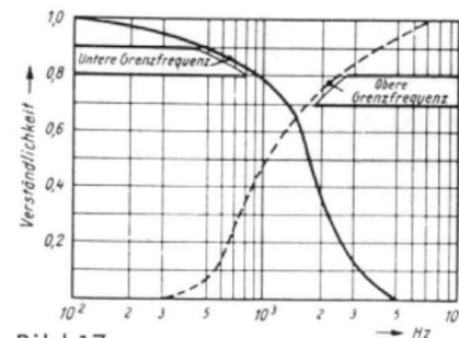
Bild 17 Verständlichkeit in Abhängigkeit von dem übertragenen Frequenzband
