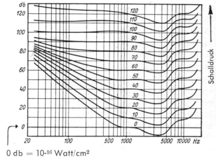
Bild 11 Kurven gleicher Lautstärkeempfindung
