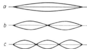
Bild 10 Zusammensetzung mehrerer sinusförmiger Tonschwingungen zum Klang. a) Grundton, b) und c) Oberschwingungen = (Vielfache vom Grundton)
