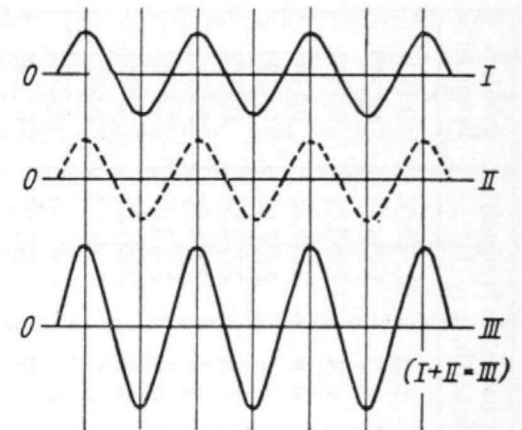
Bild 7 Interferenz zweier Wellen gleicher Länge und gleicher Phase
