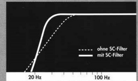
Einfluß der SC-Technik auf den Baß-Frequenzgang einer Box
