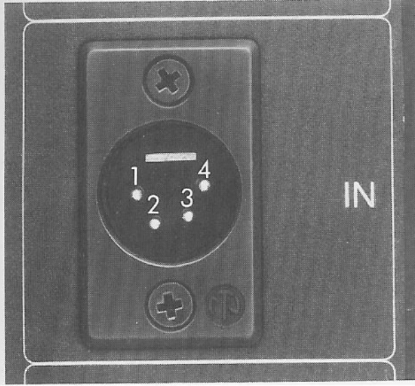
Abb. 1 Canon-Buchse der CA-Lautsprecher Belegung: 1 = Masse, 2 = linker Kanal, 3 = rechter Kanal, 4 = Steuerungspannung 15 V
