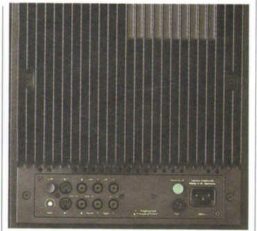
Im oberen Bild die Endstufe, darunter das Anschlußfeld einer Aktivbox.
