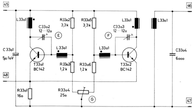
Stromlaufplan Oszillator
