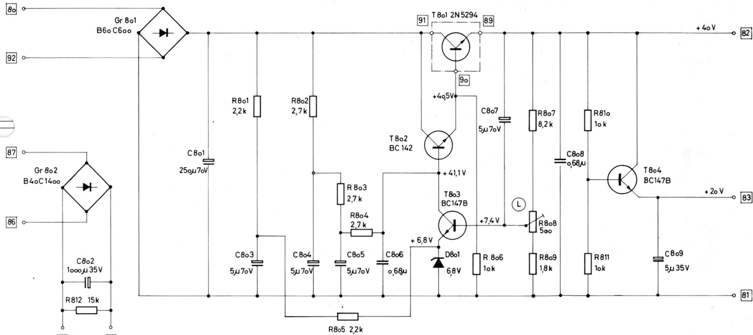
Stromlaufplan Netzteilplatte
