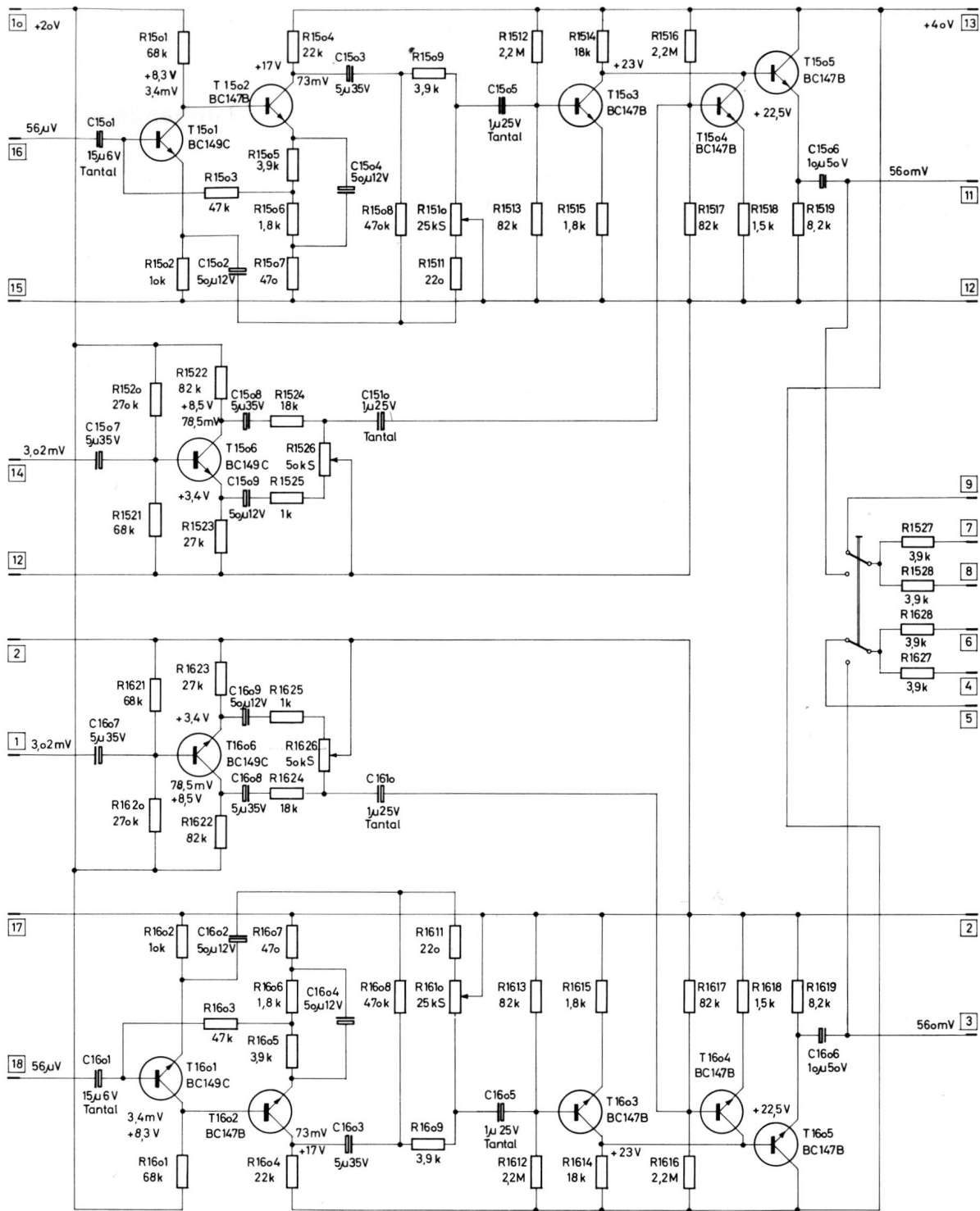
Stromlaufplan Potentiometerbaustein
