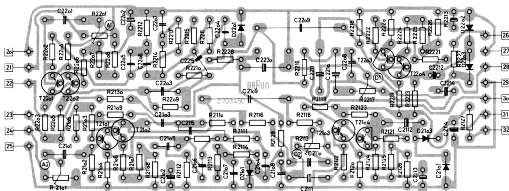
Gedruckte Schaltung, Aufspeechverstärker Leiterseite
