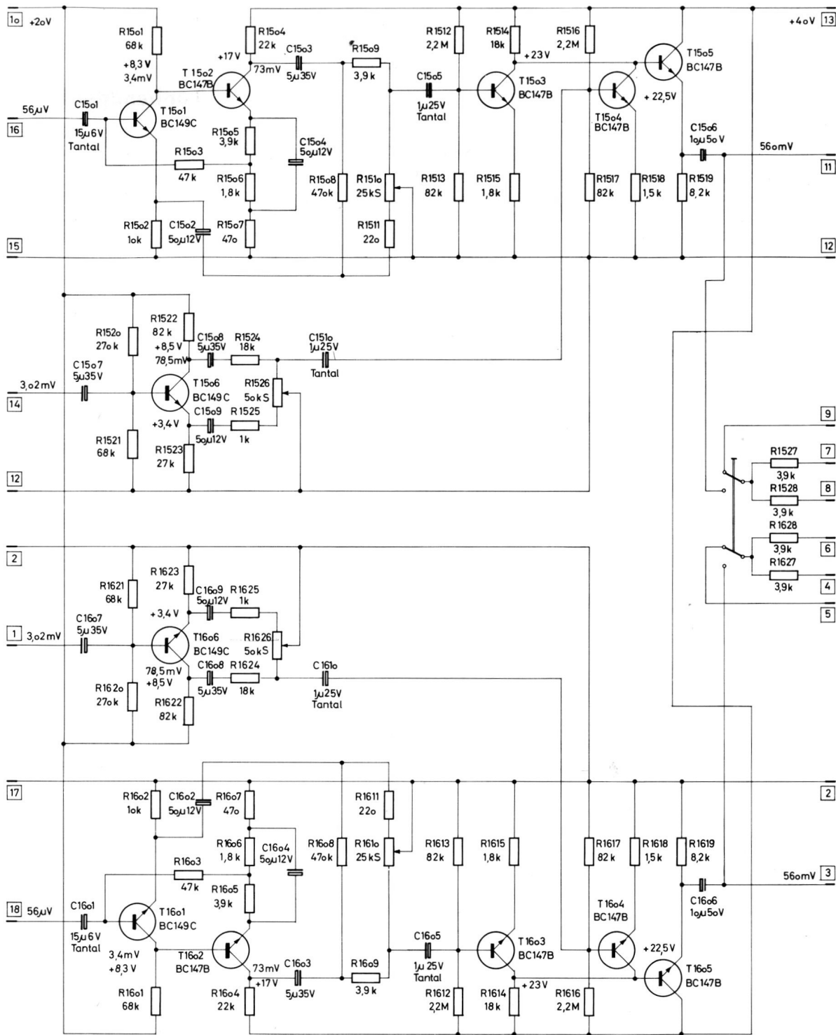
Stromlaufplan Potentiometerbaustein
