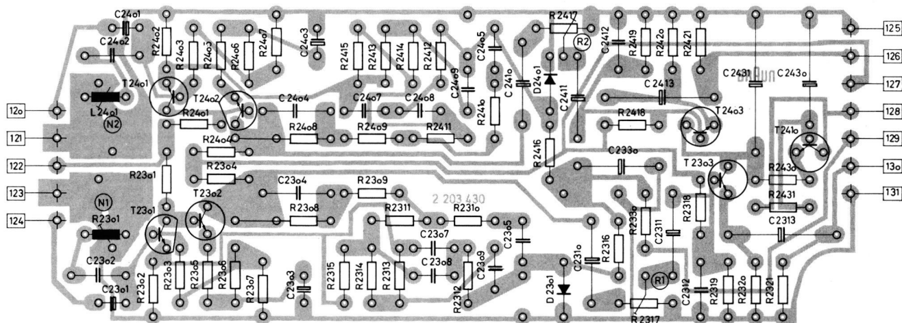
Gedruckte Schaltung, Wiedergabeverstärker Leiterseite
