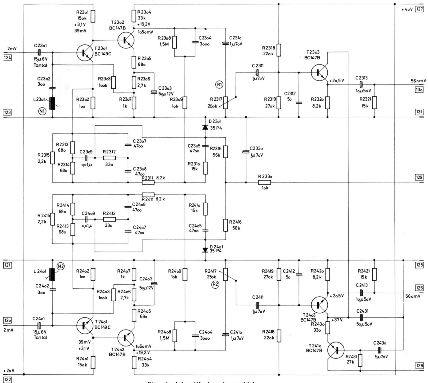
Stromlaufplan Wiedergabeverstärker
