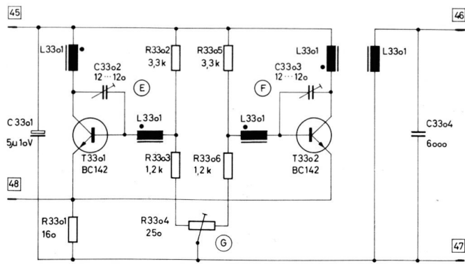
Stromlaufplan Oszillator
