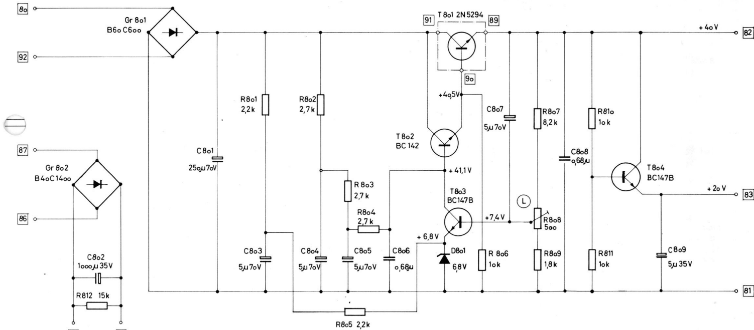
Stromlaufplan Netzteilplatte
