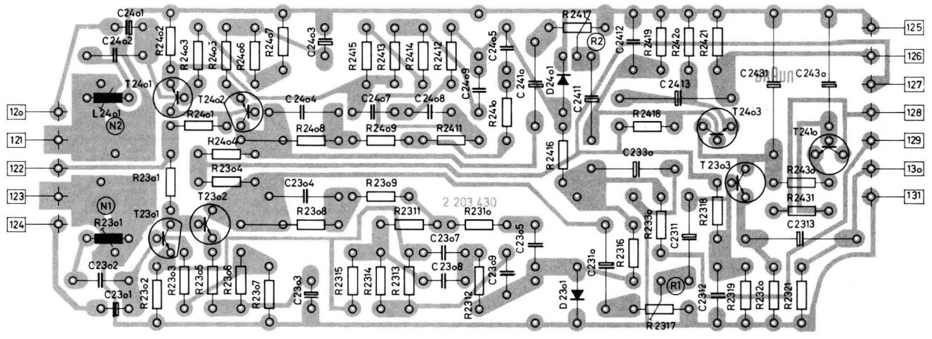
Gedruckte Schaltung, Wiedergaberverstärker Leiterseite
