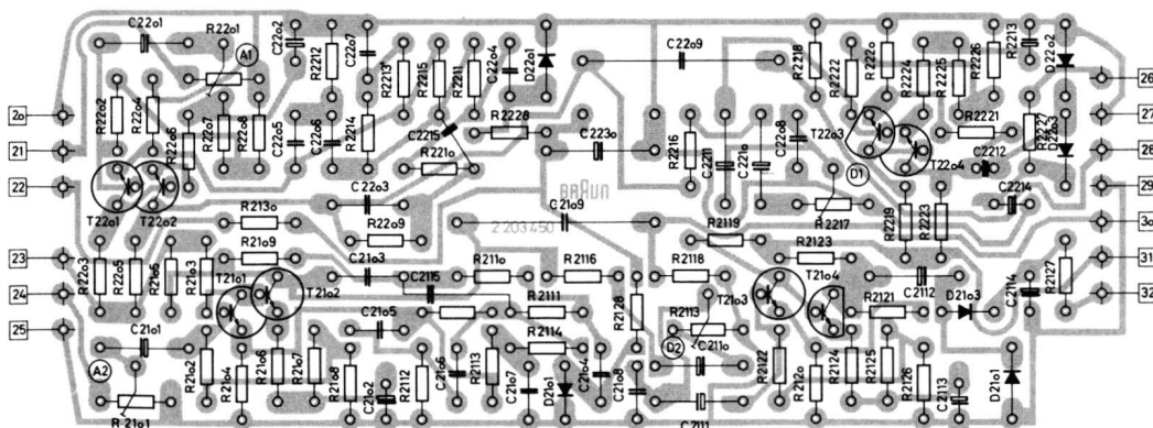
Gedruckte Schaltung, Aufsprecherverstärker Leiterseite
