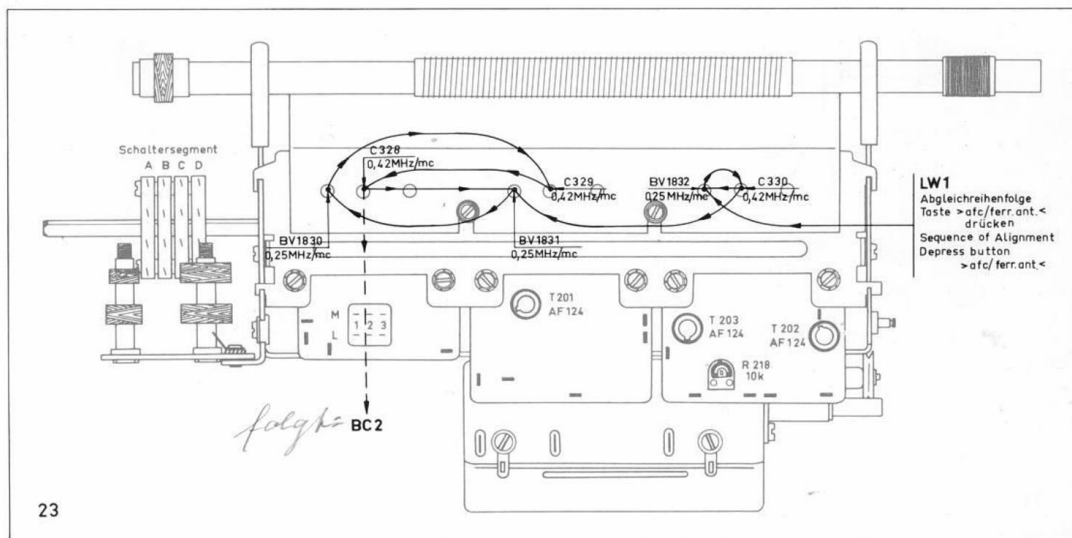
Abgleichschema LW 1
