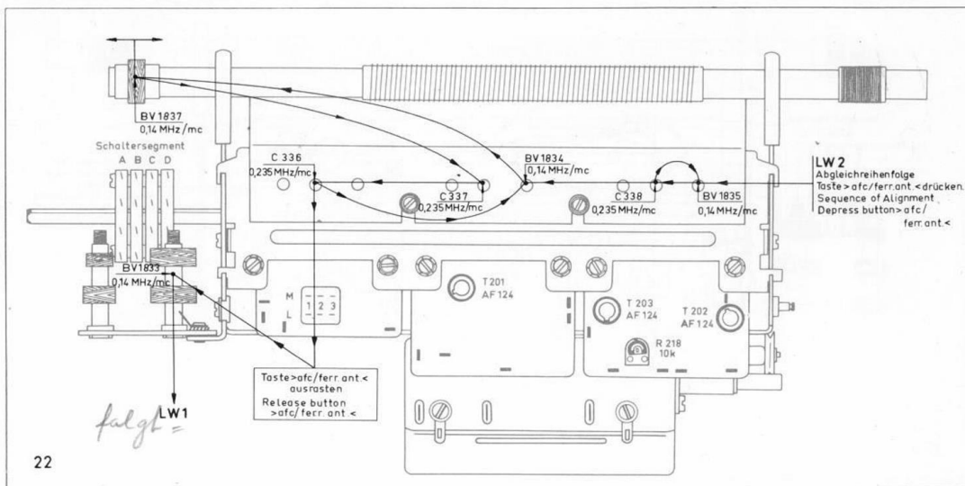
Abgleichschema LW 2
