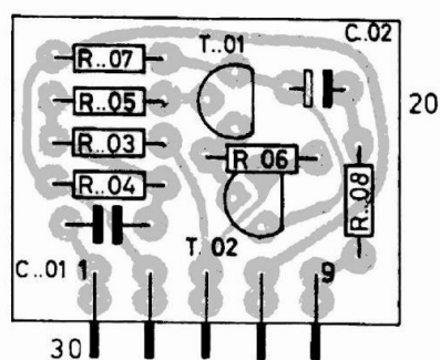
IMPEDANZWANDLER-LEITERPLATTE
