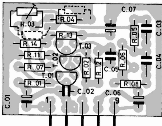
ENTZERRER-LEITERPLATTE
