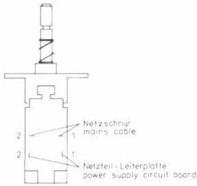
Spannungswähler voltage selector
