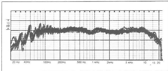
Statistisch ermittelter Frequenzgang in unserem Abhörraum
