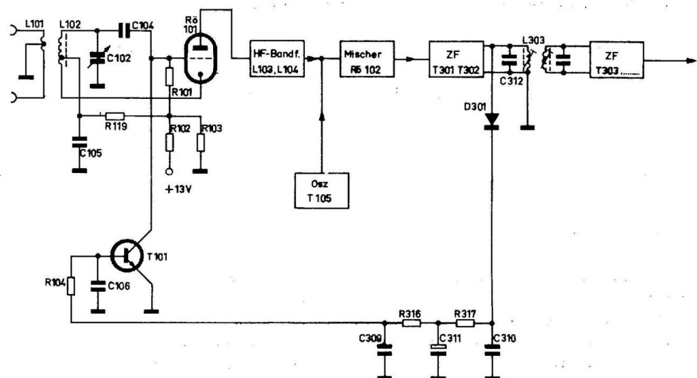
Abb. 3 Schaltungsausschnitt der automatischen Verstärkungsregelung der HF-Stufe
