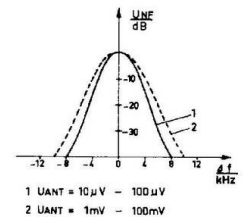
Abb. 10 Durchlaßkurve bei verschiedenen Regelzuständen bei AM-Betrieb
