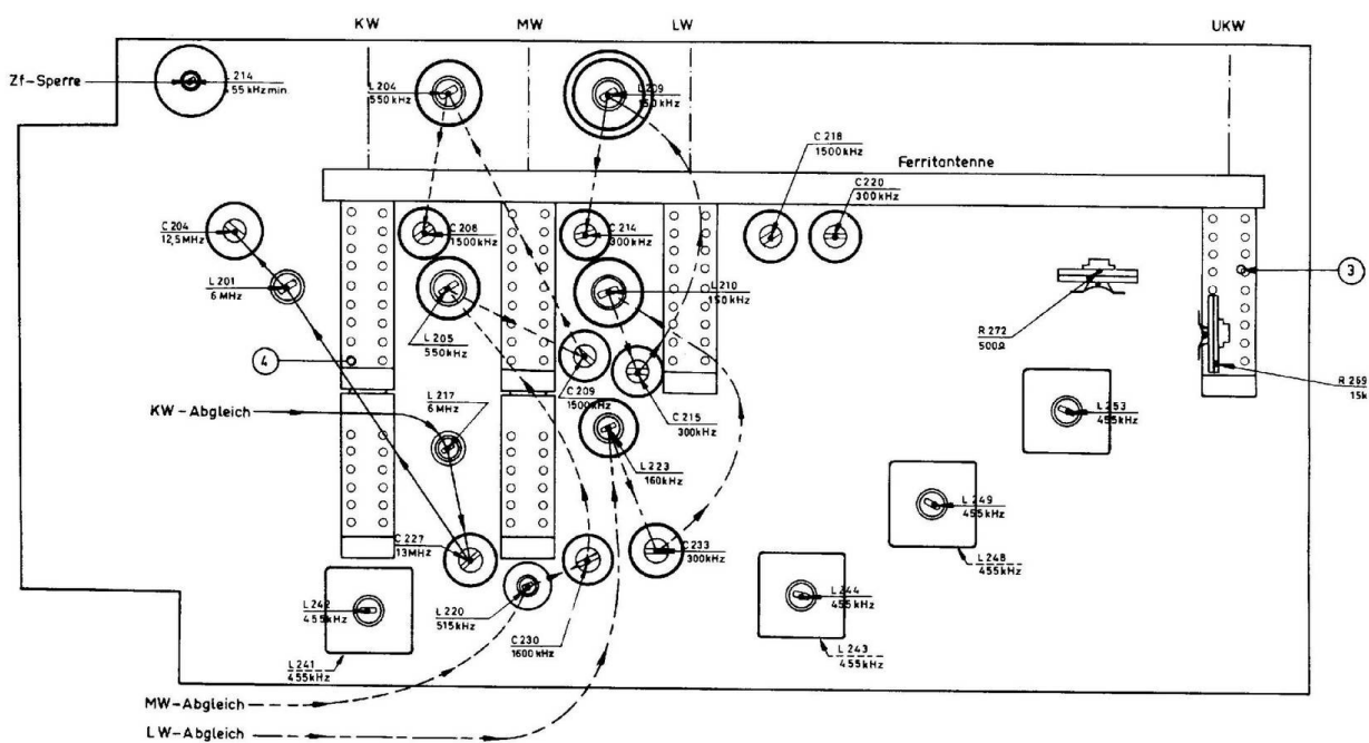
Abb. 13 Skizze zum Abgleich des AM-Teiles
