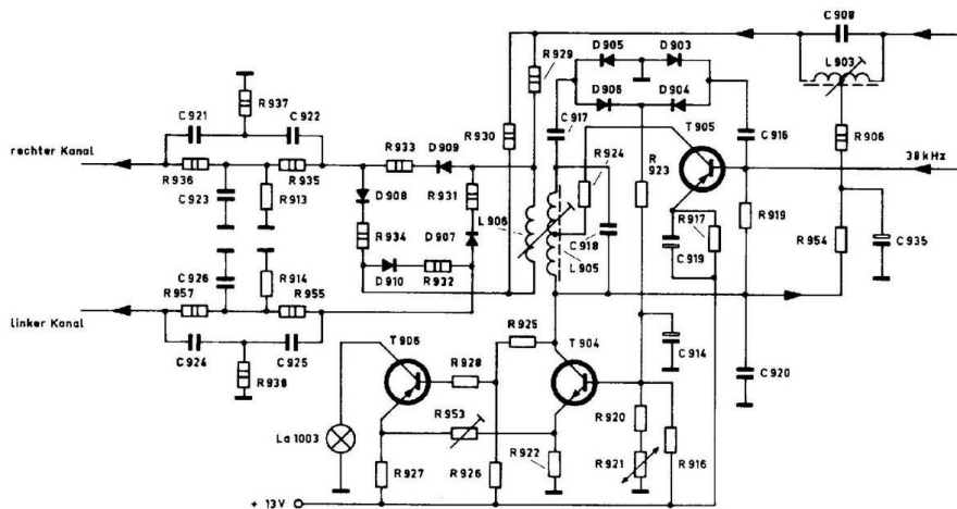
Abb. 4 Schaltungsausschnitt der Decoder-Umschaltautomatik
