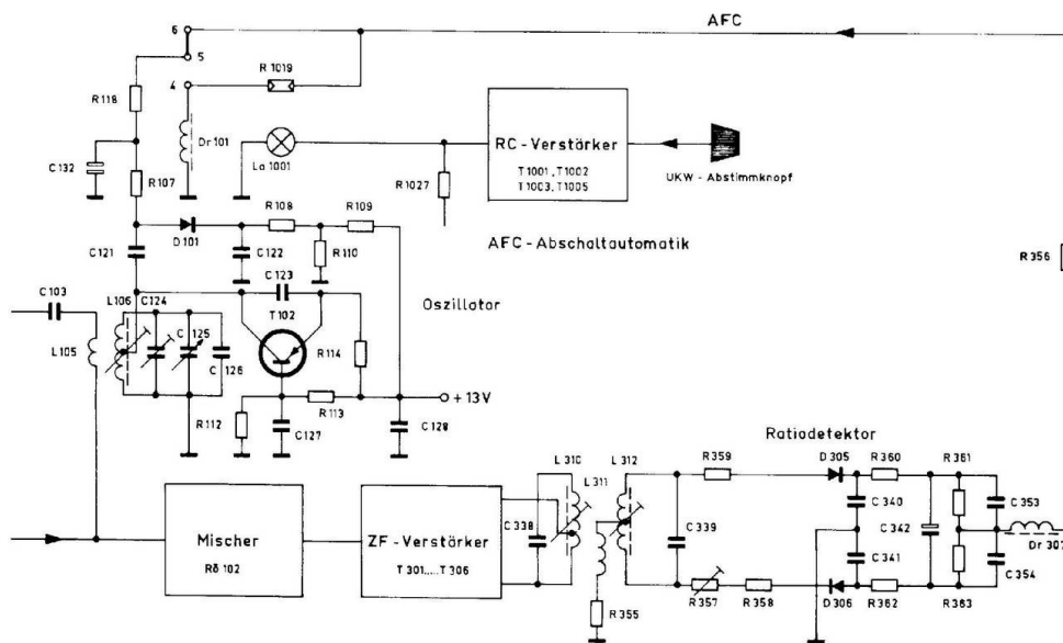
Abb. 6 Schaltungsausschnitt der AFC-Abschaltautomatik
