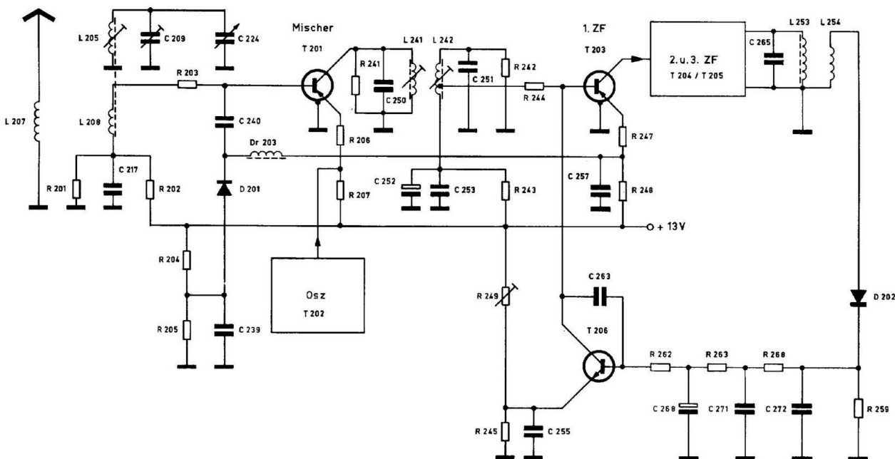
Abb. 8 Schaltungsausschnitt der automatischen Verstärkungsregelung bei AM, sh. auch Text unter 4.5.4
