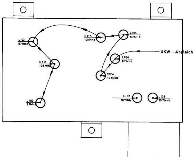
Abb. 11 Skizze zum Abgleich des UKW-Bausteines
