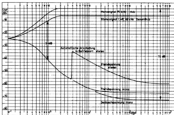
Abb. 5 Signal-Rauschkurve bei UKW-Mono- und Stereo-Betrieb NF-Ausgangsspannung als Funktion der Antennenspannung f = 90 \text{ MHz} f_{\text{mod}} = 1 \text{ kHz}
