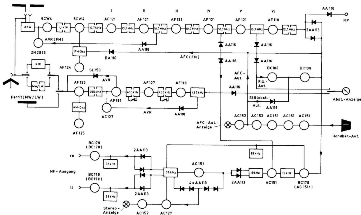
Abb. 1 Blockschaltbild
