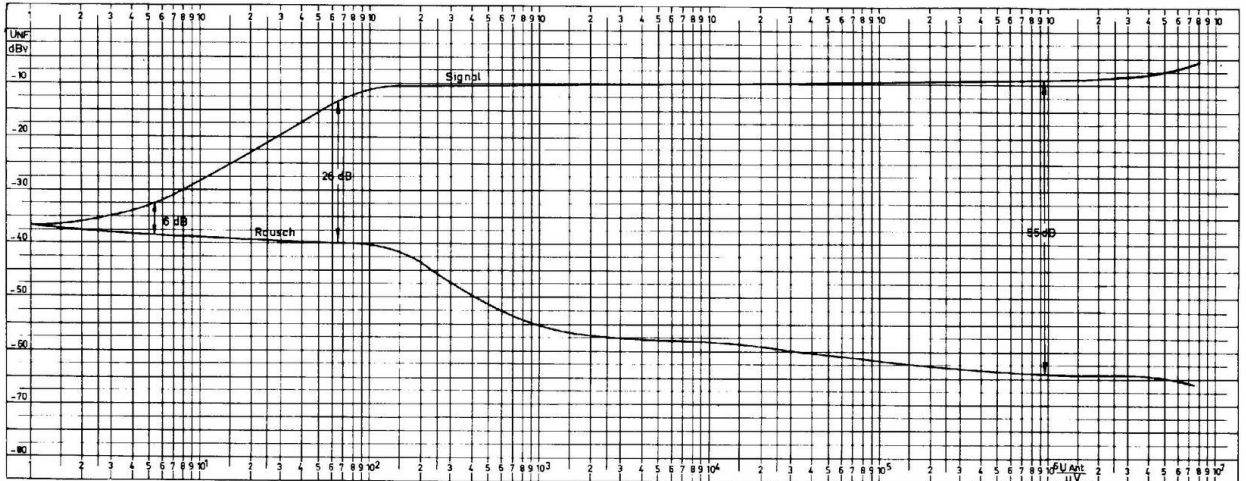
Abb. 9 Signalrauschkurve bei MW
