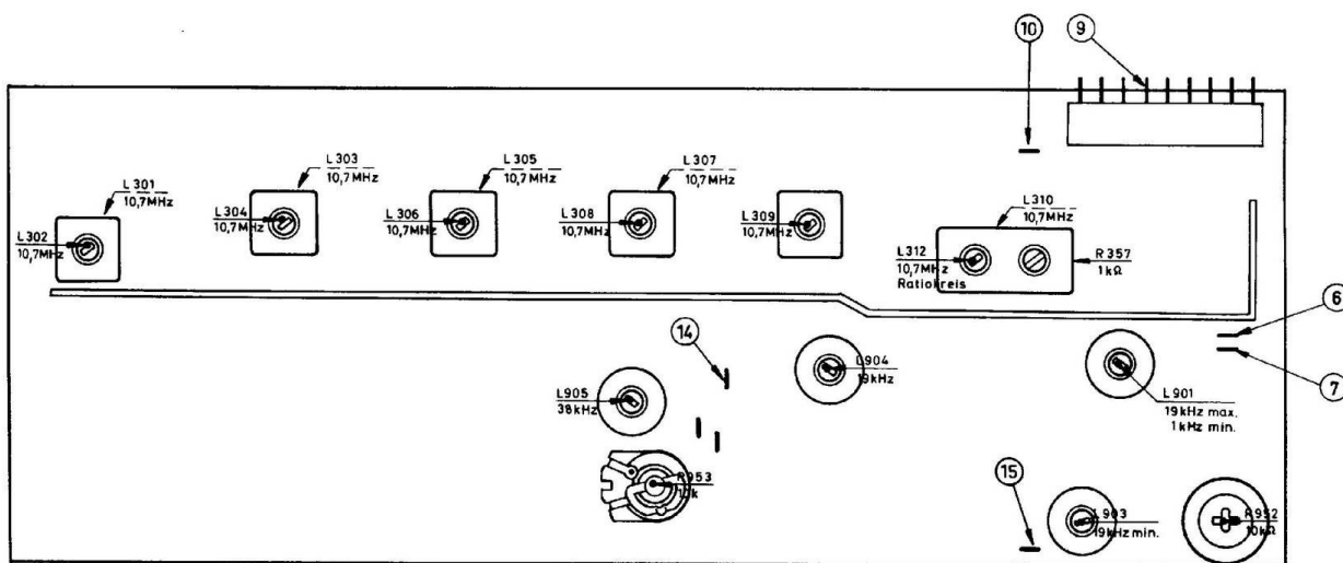
Abb. 12 Skizze zum Abgleich des FM-ZF-Verstärkers und Stereodecoders
