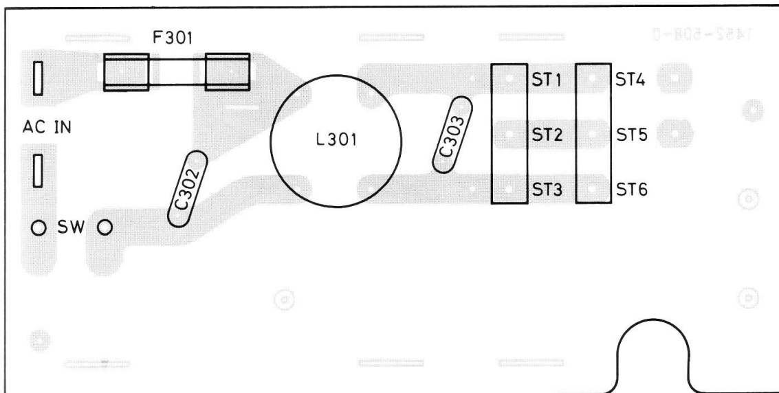
NETZTEIL - LEITERPLATTE ( Bestückungsseite )
