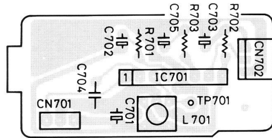
IR - EMPFÄNGER - LEITERPLATTE ( Lötseite )
