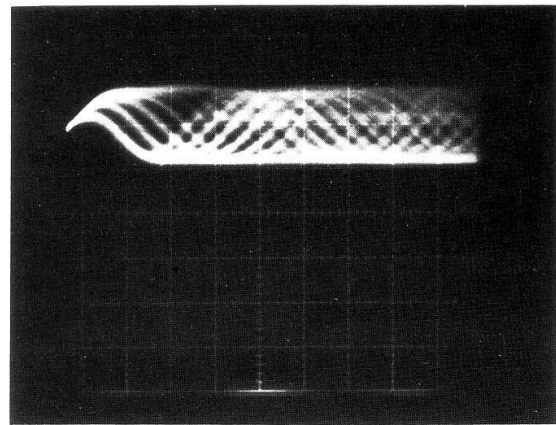
Beispiel: Schlechtes Eye - Pattern - Signal
