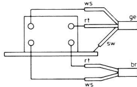
Tonkopflotanschlüsse head solder tags
