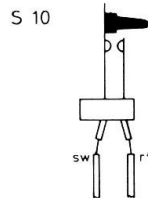
Schalterstellung bei eingelegter Cassette „Gerät eingeschaltet“ switch solder tags indicated position „cassette inserted“
