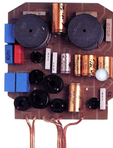
Die Frequenzweiche der CM 7 mit 4-mm 2 Innenverkabelung.
