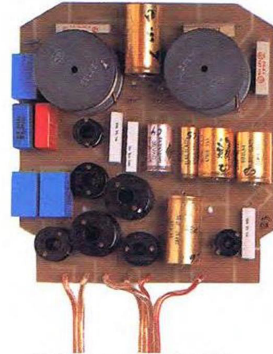
Die Frequenzweiche der CM 7 mit 4-mm-Innenverkabelung.
