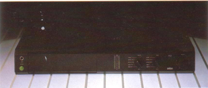
Verstärker A 2. Hochleistungsverstärker nach dem "Rail-switching"-Prinzip mit 2 x 120/180 Watt.
