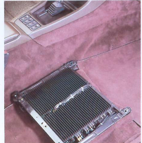
Beifahrersitz Porsche 928.
