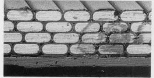
Braun Formband-Spule: 30% mehr Kraft durch 30% höhere Wicklungsdichte.
