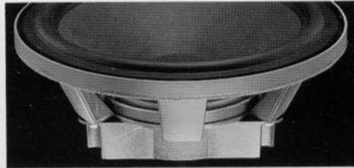
Braun Tieftöner mit "Stiffliite" Membran und verwindungssteifem Druckguß-Chassis mit guter Wärmeabteilung für hohe Belastbarkeit.
