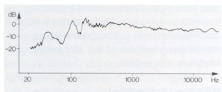
Frequenzgang einer Lautsprechereinheit (L 500/1); oben: im Freifeld, unten: im Wohnraum gemessen.
