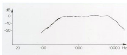
Frequenzgang eines Kalotten-Mitteltoners.
