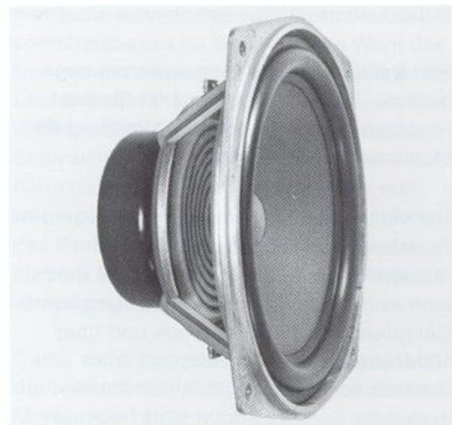
Braun Tiefton-Lautsprecher 210 mm Ø.
