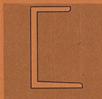
Gestellfuß Mit Verbindungsplatten kombinierbar zu Gestellsystem für Abspiel- und Steuergeräte. Verbindungsplatten beidseitig montierbar. Abmessungen: Höhe 51 cm, Tiefe oben 28 cm, unten 33,5 cm.
