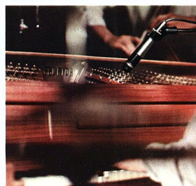
Klavier: Bei geöffnetem Deckel wird das Mikrofon ca. 40 cm über dem Klavier auf die Dämpfer in Höhe der mittleren Oktavsaiten gerichtet.
