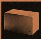
L 500/1 Zweiwegbox, für Verstärker von 10 bis 35 W, zur Regalaufstellung. Nettovolumen 15 l. Baß bis 30 Hz. Abmessungen (B, H, T): 45×25×22 cm. Gewicht 8,0 kg. Gehäuse weiß oder nußbaum.
