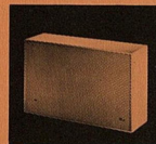
L 310 Zweiwegbox, für Verstärker von 5 bis 25 W, zur Wandaufhängung oder Regalaufstellung. Nettovolumen 7 l. Baß bis 40 Hz. Abmessungen (B, H, T): 40×25×12 cm. Gewicht 4,7 kg. Gehäuse weiß oder nußbaum. Vorrichtungen zum Hängen.
