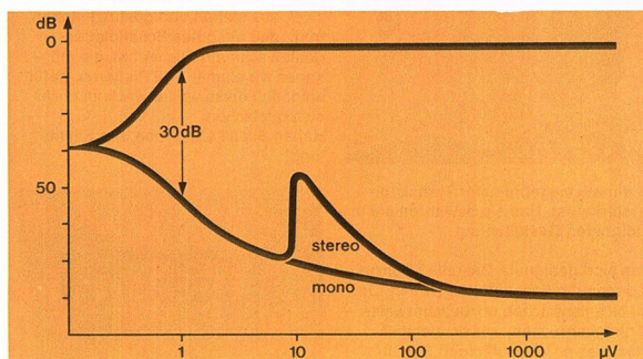
An Signal-Rausch-Kurven von Tunern läßt sich ablesen, wie beim Rundfunkempfang mit wachsender Antennen-Eingangsspannung der Fremdspannungsabstand (Rauschabstand) wächst.
