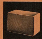
L 420/1 Zweiwegbox, für Verstärker von 10 bis 30 W, zur Regalaufstellung. Nettovolumen 6,4 l. Baß bis 35 Hz. Abmessungen (B, H, T): 32×21×17 cm. Gewicht 5,0 kg. Gehäuse weiß oder nußbaum.
