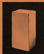
L 710/1 Dreiwegbox, für Verstärker von 20 bis 50 W, zur Regal- oder freien Aufstellung. Nettovolumen 25 l. Baß bis 25 Hz. Abmessungen (B, H, T): 31×55×24 cm. Gewicht 15,0 kg. Gehäuse weiß, schwarz oder nußbaum. Vorrichtungen zum Hängen und zur Befestigung von Fußgestellen.
