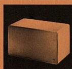
L 620/1 Dreiwegbox, für Verstärker von 20 bis 50 W, zur Regalaufstellung. Nettovolumen 15 l. Baß bis 28 Hz. Abmessungen (B, H, T): 45×25×22 cm. Gewicht 11,4 kg. Gehäuse weiß, schwarz oder nußbaum.
