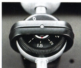
Die Auflagekraft des Tonabnehmersystems wird an einem kalibrierten Ring eingestellt.
