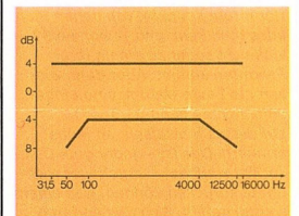
Aus DIN 45500: Toleranzfeld für den Lautsprecher-Frequenzgang.
