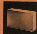
L 480/1 Zweiwegbox, für Verstärker von 10 bis 30 W, zur Wandaufhängung oder Regalaufstellung. Nettovolumen 7,9 l. Baß bis 33 Hz. Abmessungen (B, H, T): 47×28×10,5 cm. Gewicht 5,7 kg. Gehäuse weiß oder nußbaum. Vorrichtungen zum Hängen.
