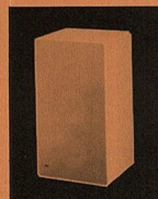
LV 720 Dreiwegbox mit eingebauten Endverstärkern, für Vorverstärker von 0,39 bis 2,45 V Ausgangsspannung. Zur freien Aufstellung. Nettovolumen 22 l. Baß bis 25 Hz. Maximaler Schalldruck 107 dB in 1 m Entfernung. Verstärkerleistungen 60/20/20 W. Klirrfaktor 0,1%. Abmessungen (B, H, T): 31×55×26 cm. Gewicht 18 kg. Gehäuse weiß oder nußbaum. Vorrichtung zur Befestigung von Fußgestellen.
