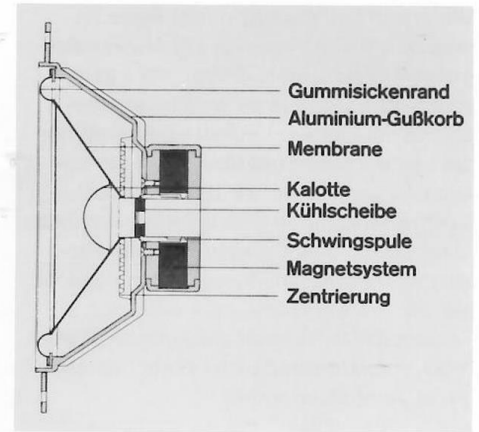
Aufbau eines dynamischen Lautsprechersystems (Tieftöner).
