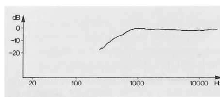
Frequenzgang eines Kalotten-Hochtöners.
