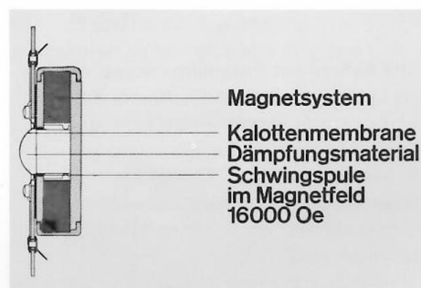
Aufbau eines Hochton-Lautsprechers mit Kalottenmembran.
