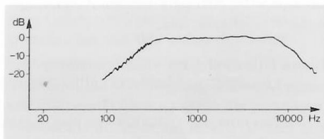
Frequenzgang eines Kalotten-Mitteltöners.
