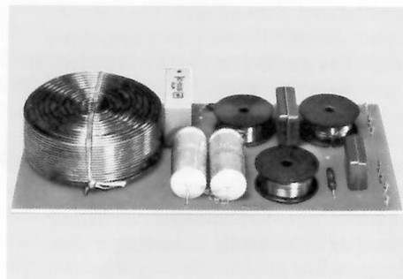
Frequenzweiche einer Dreiweg-Box (L 620/1).
