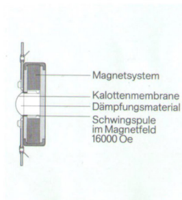
Schnitt durch einen Kalottenhochton-Lautsprecher
