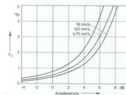
Aussteuerungskennlinie
