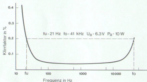
Leistungsbundbreite des CSV 300
