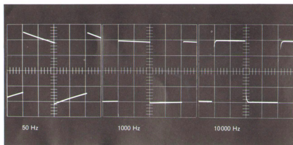
Wiedergabe von Rechteckimpulsen bei verschiedenen Frequenzen
