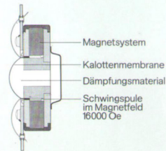
Schnitt durch einen Kalotten-mittelton-Lautsprecher.
