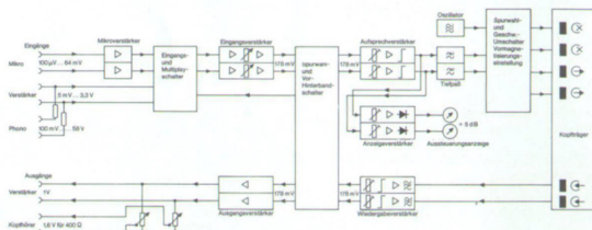
Blockschaltbild des NF-Teils
