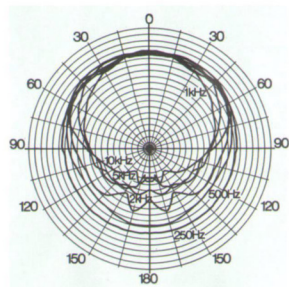
Richtcharakteristik bei verschiedenen Frequenzen
