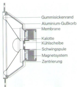
Schnitt durch den Tieftonlautsprecher
