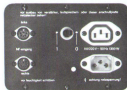
Rückseitige Anschlußplatte
