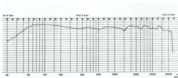
Frequenzgang der Lautsprechereinheit
