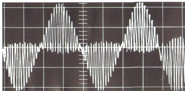
Oszillogramm eines UKW-Stereo-Signals
