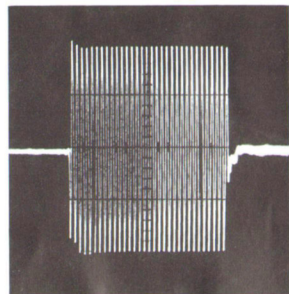
Impulsverhalten des Kalottenhochton-Lautsprechers bei einer Frequenz von 5 kHz
