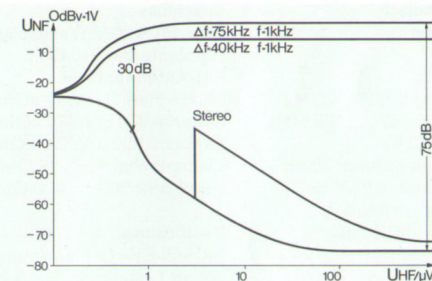
Signal-Rauschverhältnis des Tuners bei 100 MHz
