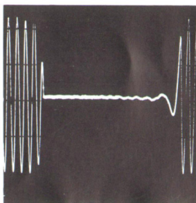
Impulsverhalten des Tieftonlautsprechers
