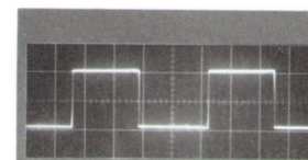
Rechteck-Verhalten des Verstärkers
