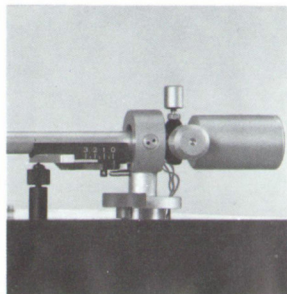
Tonarmlagerung mit Einstell-skala für die Auflagekraft
