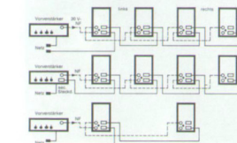
Anschlußmöglichkeit mehrerer LV 1020
