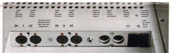
Beim audio (und bei den studio-Geräten) liegen alle Anschlüsse versenkt in der Bodenplatte. Die Rückseite des Gerätes bleibt frei von Steckern.
