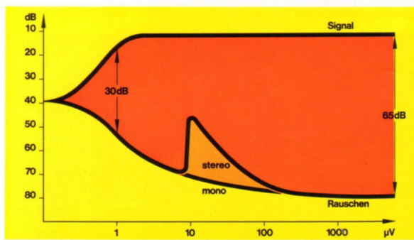
An Signal-Rausch-Kurven (hier von Braun Tunern) läßt sich ablesen, wie beim Rundfunkempfang mit wachsender Antennen-Eingangsspannung der Fremdspannungsabstand (Rauschabstand) wächst.
