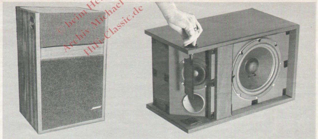
Eine Direct-Reflecting-Box für jedermann. Die Regal-Box Bose 301. Über einen einstellbaren Reflektor kann die hochfrequente Schallenergie auf reflektierende Flächen gelenkt werden
