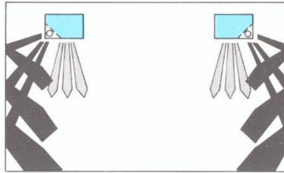
Direkt/Indirekte Abstrahlung: Der Schlüssel für richtige Stereowiedergabe.
