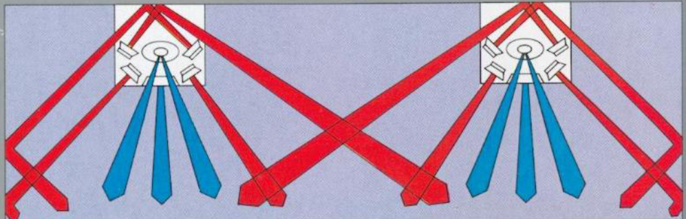
Die Abstrahlcharakteristik des BOSE 601 Direct/Reflecting Lautsprechersystems.
