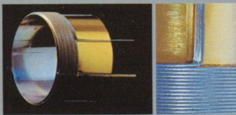
Die Helical-Schwingspule. Rechteckiger Aluminiumdraht wird in einer Lage hochkant auf den Spulenkörper gewickelt. Isolation und Wicklung verkräften Impulstests mit knapp 4000 Watt.
