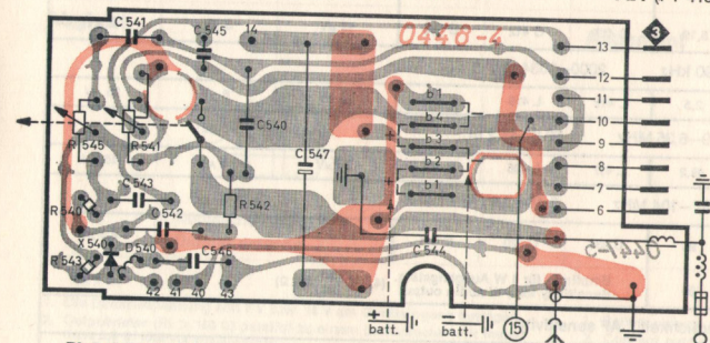
PL 5 (PT 4156/11z) Bestückungsseite / Components side
