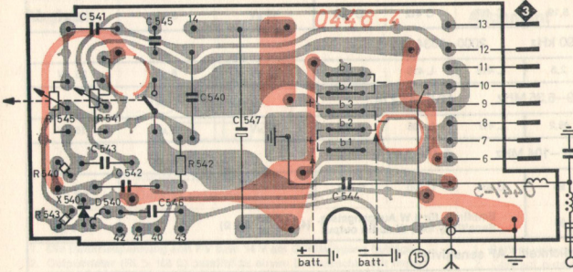
PL 5 (PT 4156/11z) Bestückungsseite / Components side
