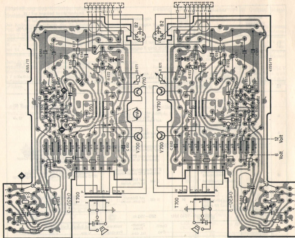
PL 7 (PT 4155/11z) Bestückungsseite / Components side
