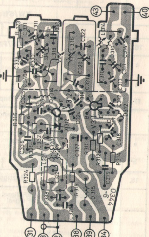
PL 6 (PT 4157/01z) Bedruckungsseite / Printed side
