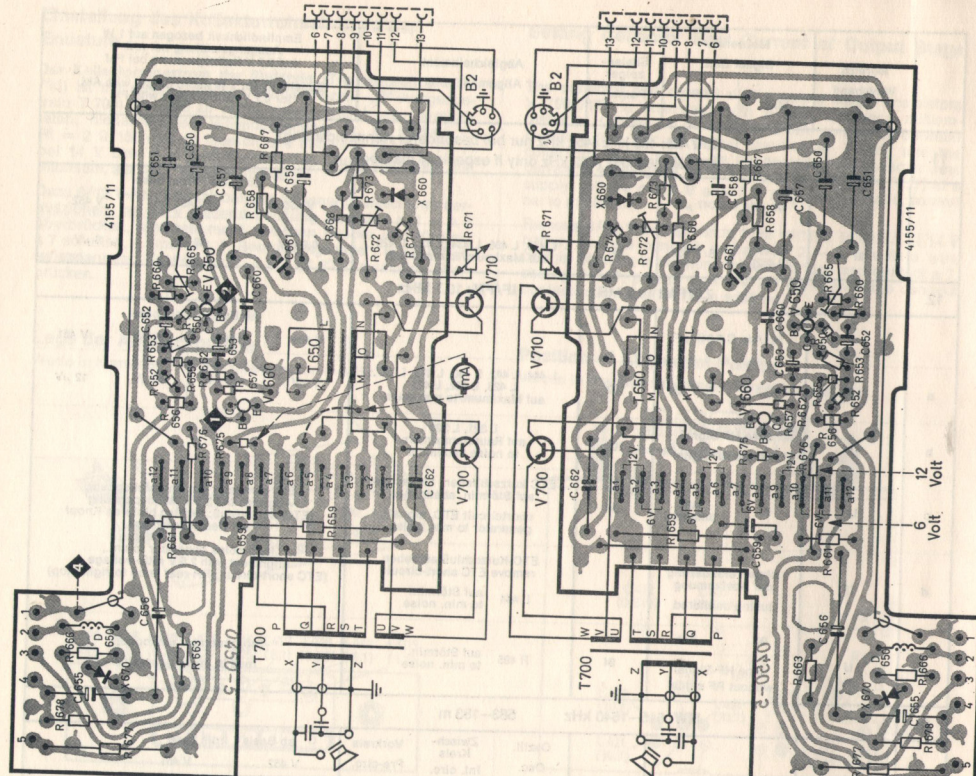
PL 7 (PT 4155/11z) Bedruckungsseite / Printed side
