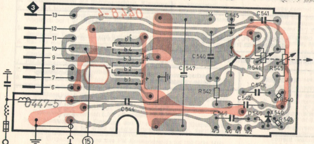
PL 5 (PT 4156/11z) Bedruckungsseite / Printed side
