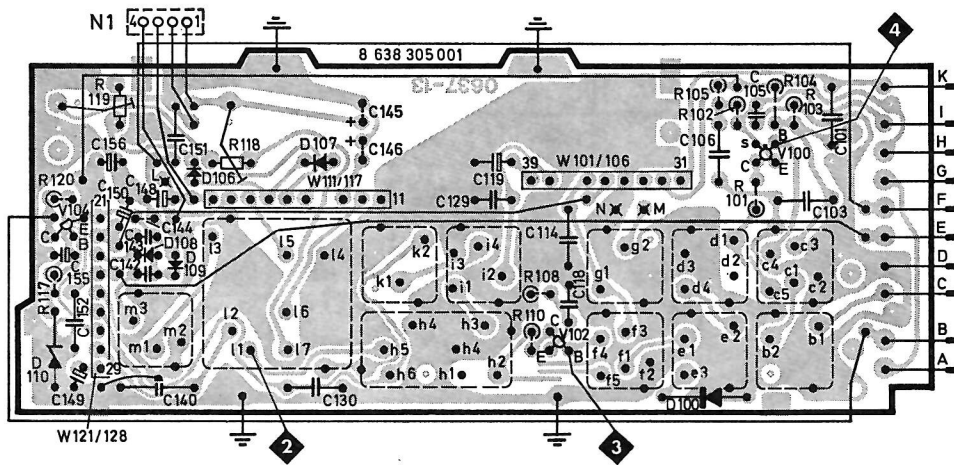
PL 1 8 638 305 001 Bedrucksungsseite / Printed side
