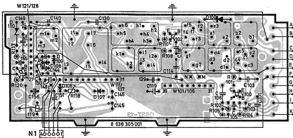
PL 1 8 638 305 001 Bestückungsseite / Components side
