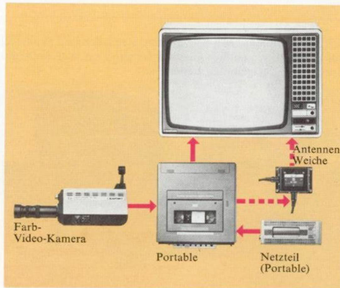
Blaupunkt VideoTechnik. Einsatzmöglichkeit Nummer drei: Portable im Heimbetrieb.
