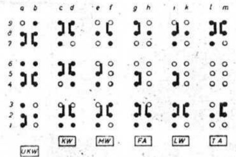
Gezeichnete Schalterstellung UKW
