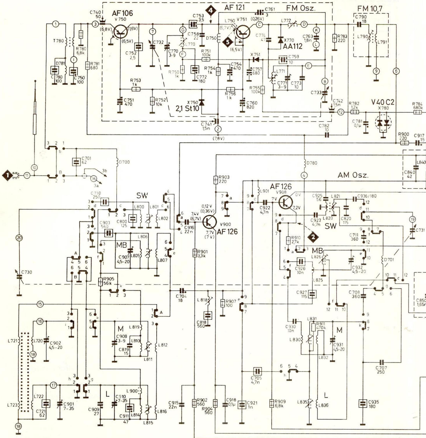
Schalterdiagramm / Switch diagram
