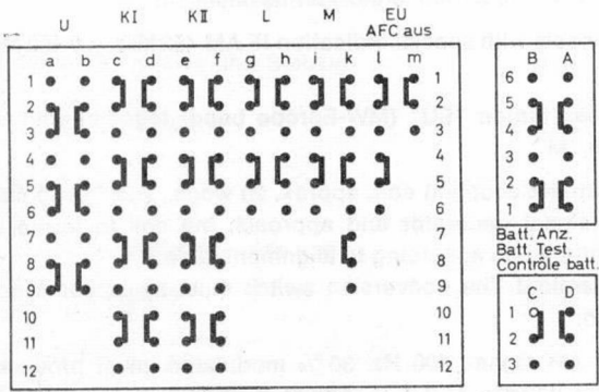
Schalterdiagramm/Switch diagram Diagramme du commutateur
