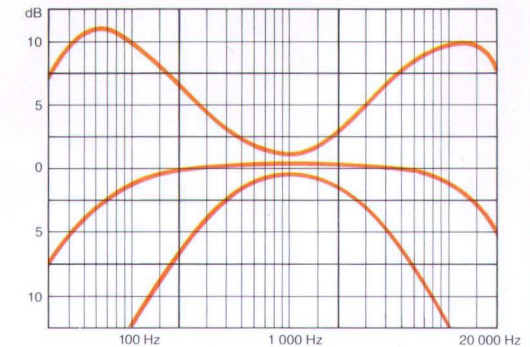
Die Regelbereiche der Höhen- und Tiefenregler.
