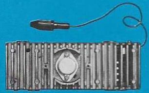
SPT 7 102 Spannungswandler 24 V auf 12 V. Minus an Masse.
