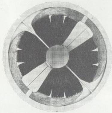
Ablenkspule für konventionelle Dickhals-Röhre (Sattel-Spule)
