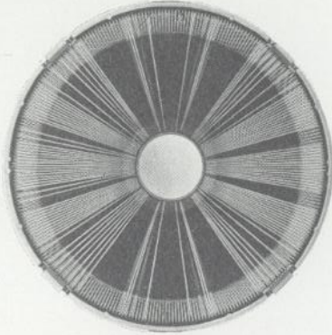
Toroid-Ablenk-Spule für Dünnhals-Röhre (Blaupunkt) Symmetrischer Aufbau = gleichbleibende Konvergenz und Schärfe auch in Randzonen.
