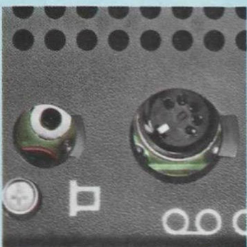
Genormte Anschlußbuchsen für Plattenspieler/Tonbandgerät und Außenlautsprecher/Kopfhörer.
