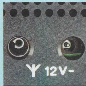
Anschlußbuchse für Außen- oder Autoantenne. Schaltbuchse für externe 12-Volt-Batterie, dazu Anschlußkabel mit Auto-Entstörung.
