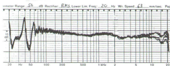
Frequenzgang B&M Beta (li.) und Sigma, auf Achse und um 40 Grad gedreht
