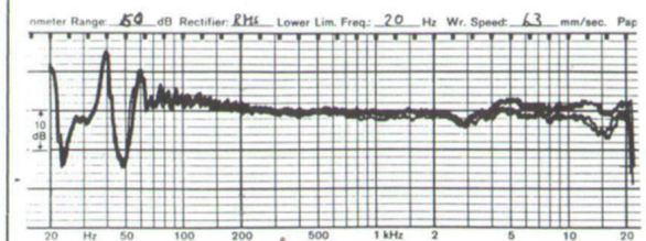
Frequenzgang B&M Beta (li.) und Sigma, auf Achse und um 40 Grad gedreht
