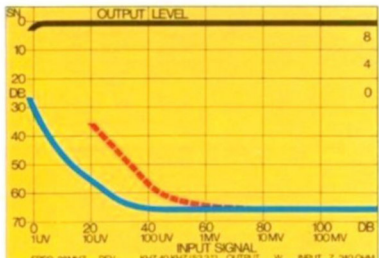
Fremdspannungsabstand (bei 50 mW/Kanal) Tape 1 (oder Keramik-Tonabnehmer)
