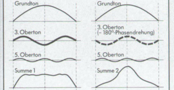
Das Bild 1 zeigt ein vereinfachtes Musiksignal (Summe 1), das sich aus dem Grundton und 2 Obertönen zusammensetzt. Bild 2 zeigt die gleichen Teilsignale mit gleicher Frequenz und Amplitude. Lediglich der 3. Oberton wurde in seiner Phase um 180° gedreht. Das resultierende Musiksignal (Summe 2) ist offensichtlich ein völlig anderes.
