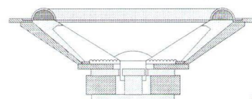
Querschnitt durch einen Tieftöner mit gewöhnlichem Membrankegel. Er ist besonders anfällig für Partial-schwingungen und hat meist ein schlechtes „roll-off“-Verhalten.
