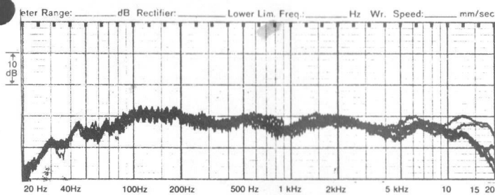
Statistisch ermittelter Frequenzgang in unserem Abhörraum
