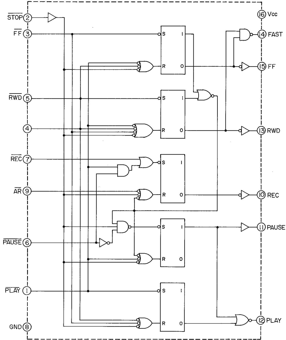
Fig. 5 M54410P
