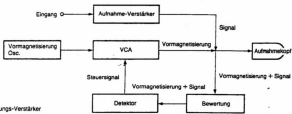
Fig.-2 Blockdiagramm des DOBLY HX PRO Systems zur Ausdehnung des Aussteuerungsmarginals
