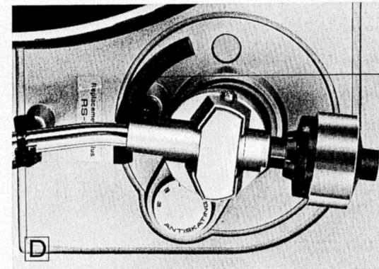
Arm Lifter Elevation Adjustment Screw Vis de réglage de hauteur du bras acoustique Höheneinstellschraube des Tonarmhebers
