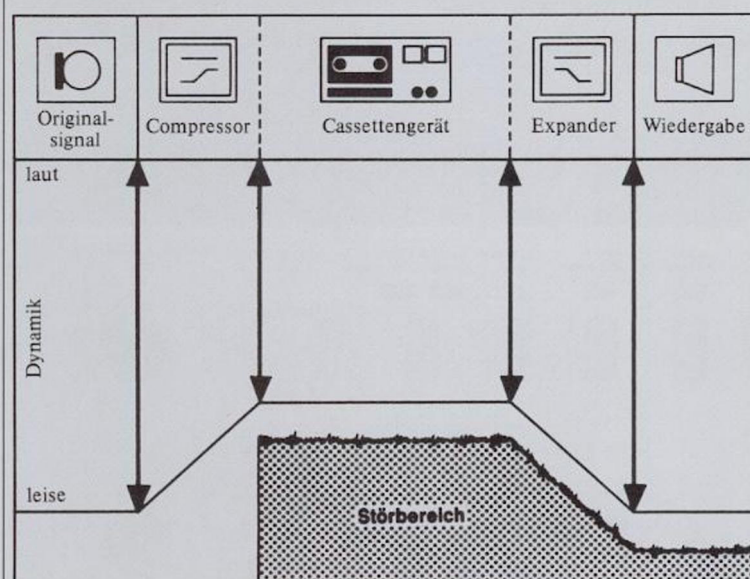
Wirkungsweise des HIGH COM-Rausch- und Störunterdrückungs-Systems
