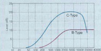
Vergleich niedrigstufiger Kodierung: NR-Systeme des Dolby B- und C-Verfahrens.
