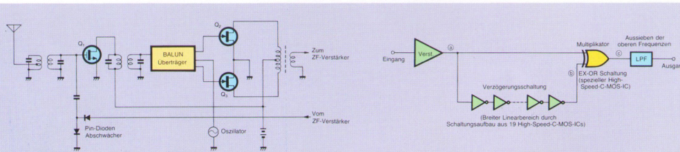
Abb. 1 Schaltbild der Eingangsstufe
