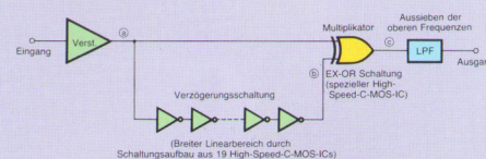
Abb. 2 Funktionsprinzip des DGL-Detektors
