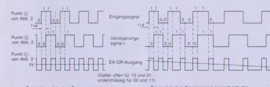
Abb. 3 Bei nicht moduliertem Eingangssignal ergibt sich ein gleichwertiger EX-OR-Ausgang und 0 am Ausgang des Tiefpassfilters. Bei moduliertem Eingangssignal spiegelt sich das Kompressionsverhältnis des Signals in der Ungleichförmigkeit des EX-OR-Ausgangs. Die am Ausgang des Tiefpassfilters anliegenden integrierte steuern, wie durch die schräg verlaufende Linie angedeutet, die Änderung des elektrischen Potentials (Nutzsignal).
