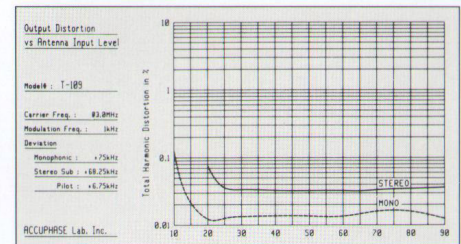
Ausgangsverzerrung versus Antennen-Eingangspegel
