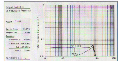
Ausgangsverzerrung versus Modulationsfrequenz
