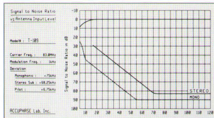
Signal/Rauschverhältnis versus Antennen-Eingangspegel
