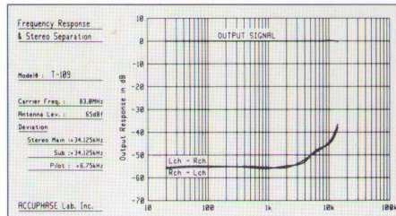
Frequenzgang und Stereotrennung
