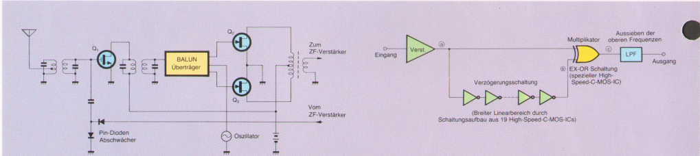
Abb. 2 Funktionsprinzip des DGL-Detektors
